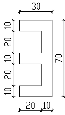
חתך א-א ק.מ. 1:20
