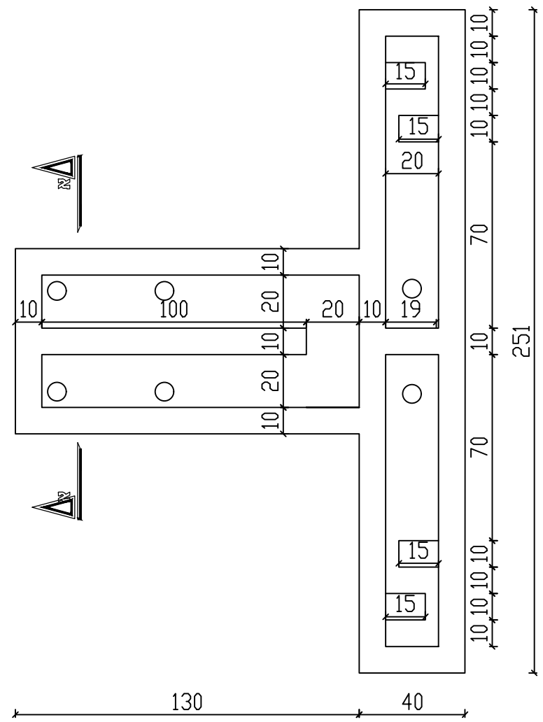
תוכנית תעלות ק.מ. 1:20
