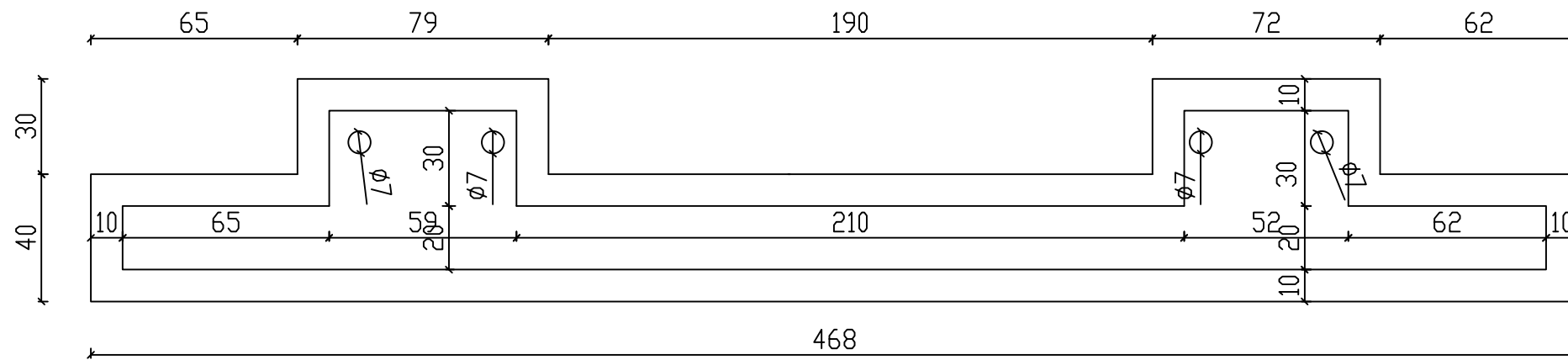
תוכנית תעלות ק.מ. 1:20
