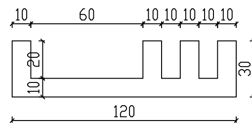
חתך ג-ג ק.מ. 1:20
